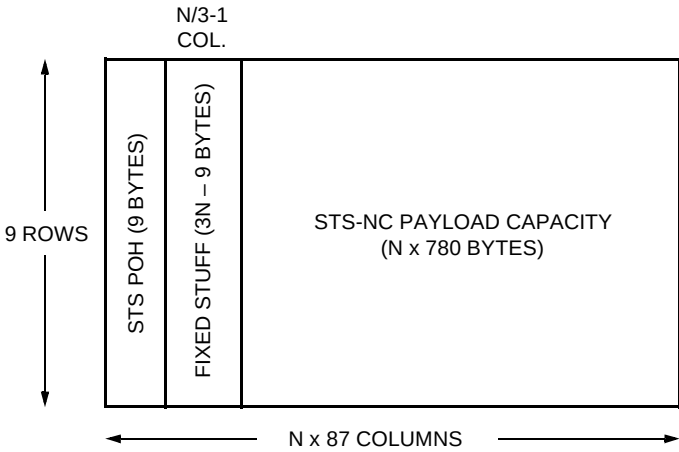
Figure 41. STS-Nc SPE
