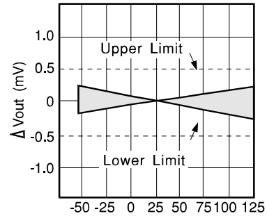
Temperature °C VRE210MA
