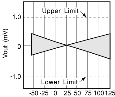
Temperature °C VRE210M
