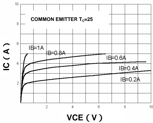
IC - VCE
