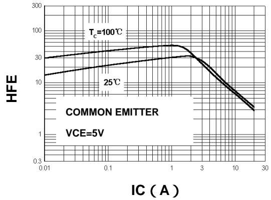
HFE - IC
