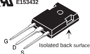
ISOPLUS247™ (IXFR) E153432
