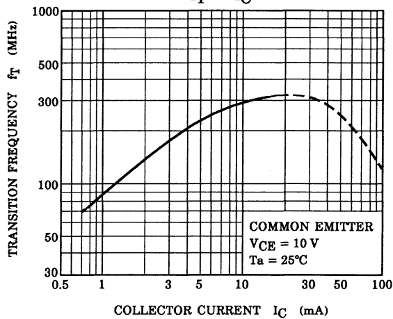
f_T - I_C
