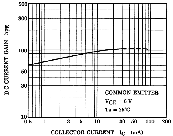
h_{FE} - I_C
