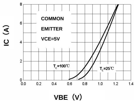
IC - VBE
