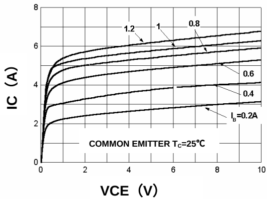
IC - VCE
