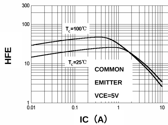
HFE - IC
