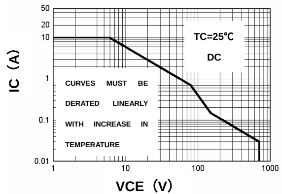
SOA
