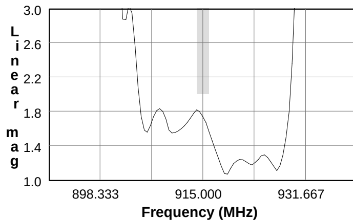
S11 VSWR
