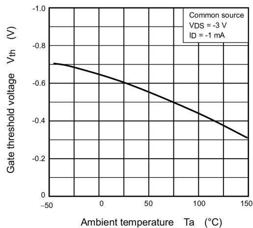
Fig. 8.7 V_{th} - T_a
