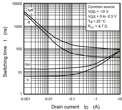
Fig. 8.11 t - I_D
