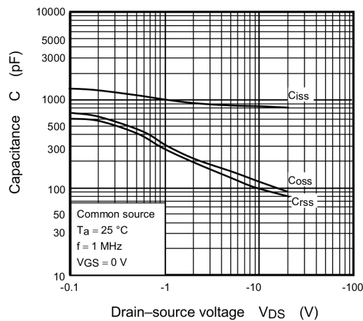
Fig. 8.9 C - V_{DS}
