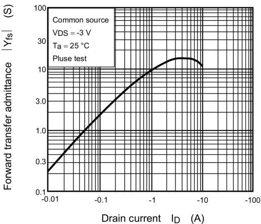
Fig. 8.8 |Y_{fs}| - I_D
