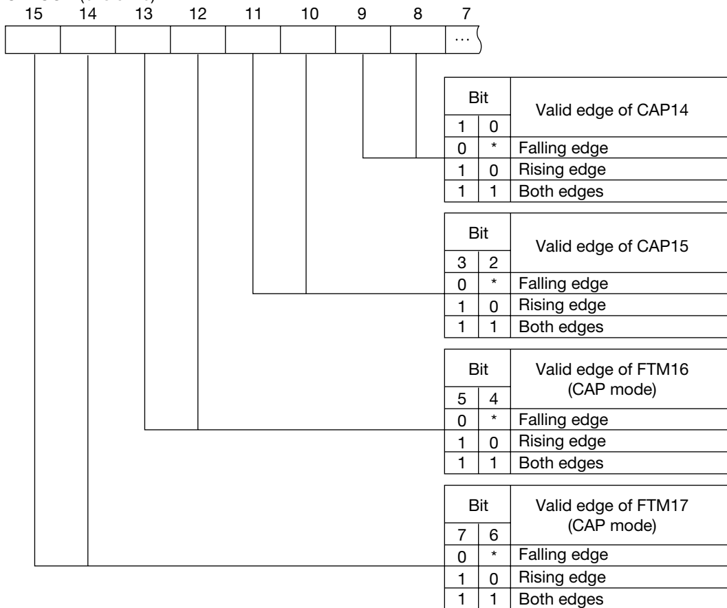
CAPCON (bits 8–15)
