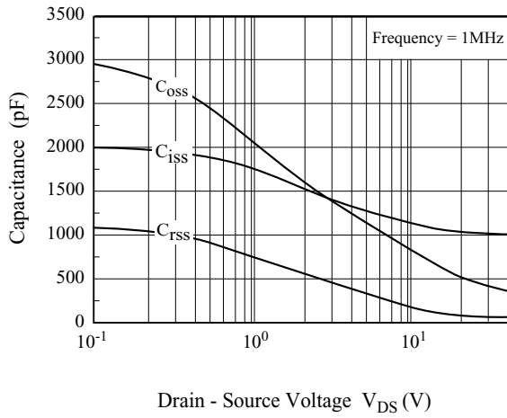
Fig 7. C - V_{DS}
