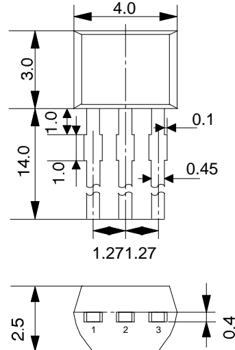
電極接続
