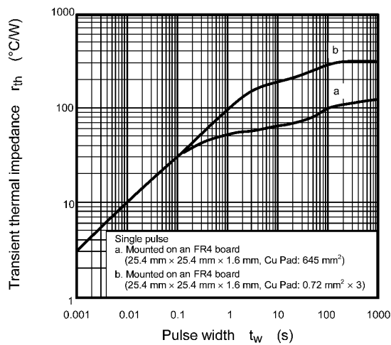
Fig. 8.11 r_{th} - t_w
