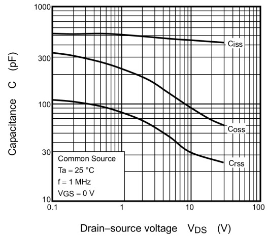
Fig. 8.8 C - V_{DS}
