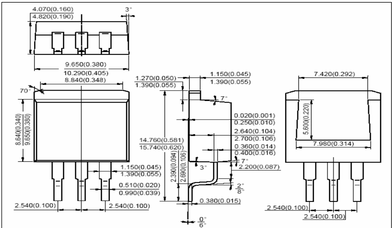
D²PAK (TO-263)
