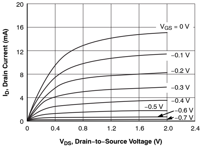
Figure 1. I_D - V_{DS}
