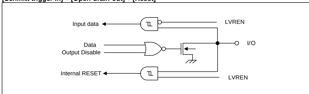
R35/RESETB
