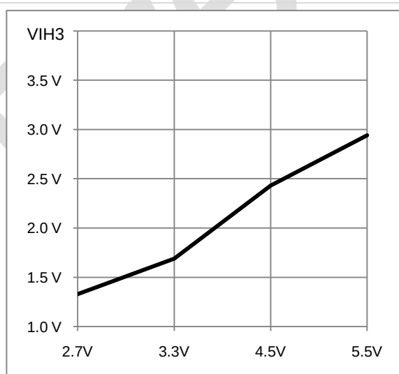
Figure 7-25 V IH3 - V DD
