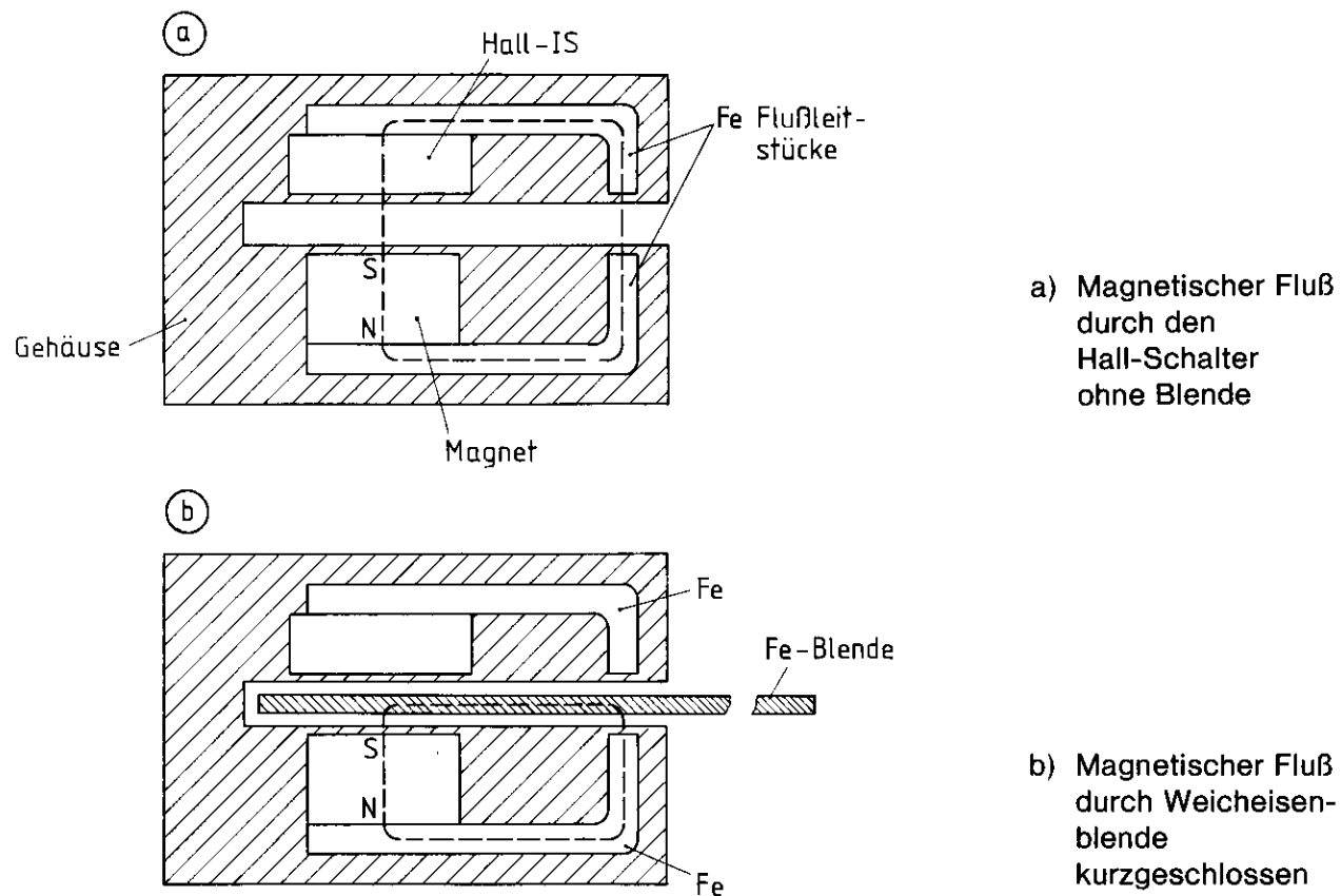
Bild 1 Funktionsprinzip
