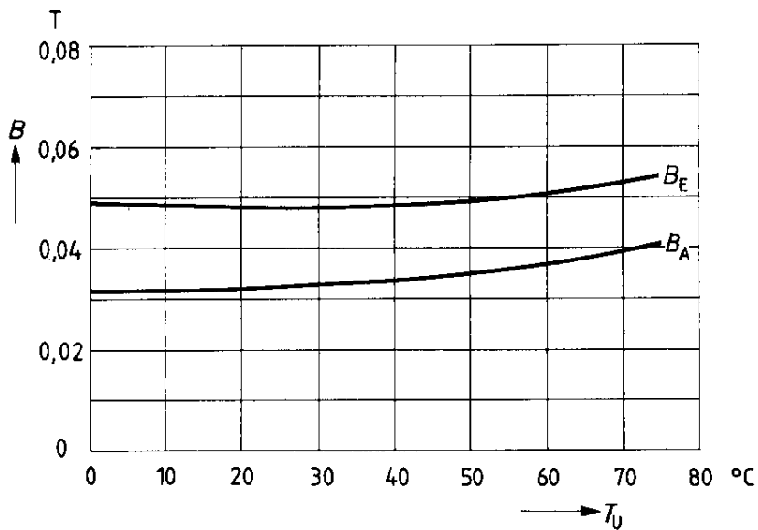
B_E, B_A = f(T_U) , typ.
