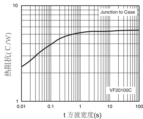
图4. 单侧热阻抗
