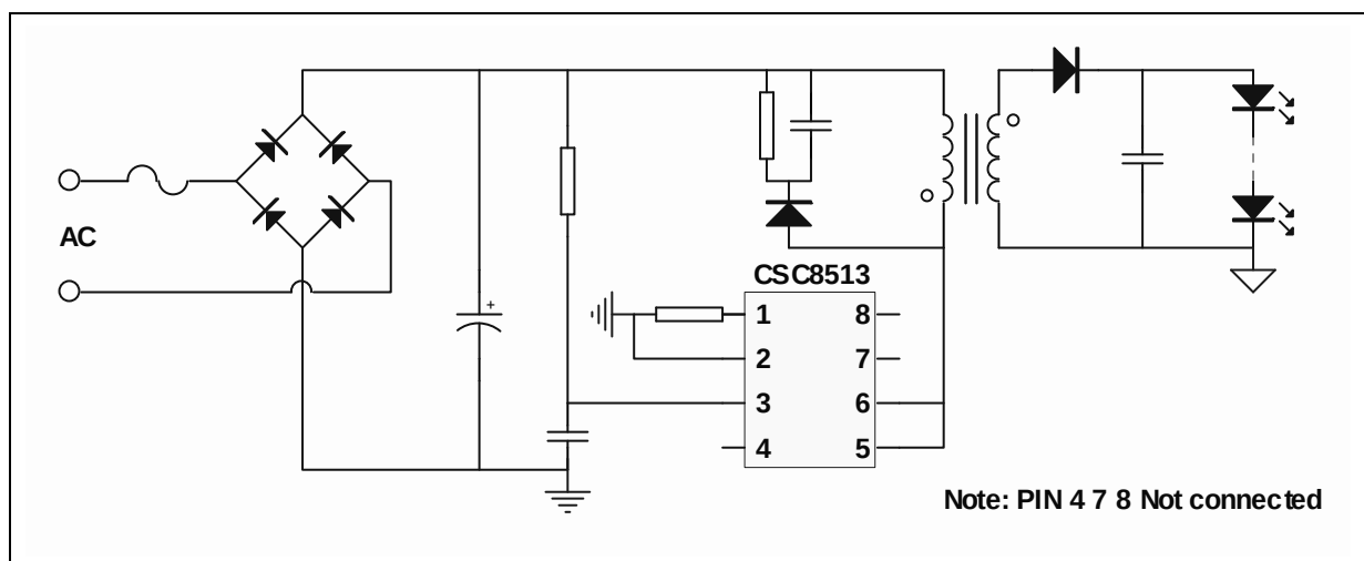
应用线路图
