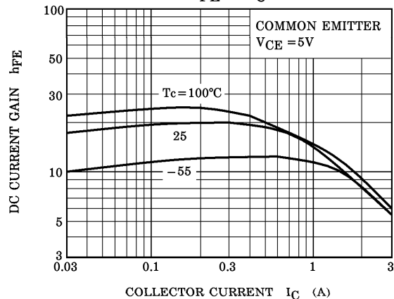
h_{FE} - I_C
