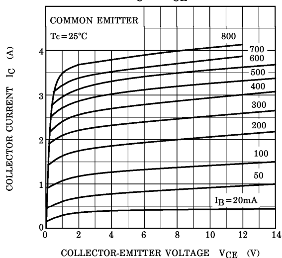
I_C - V_{CE}
