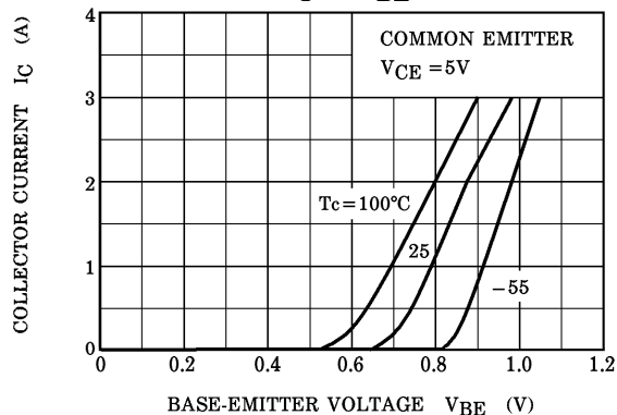
I_C - V_{BE}
