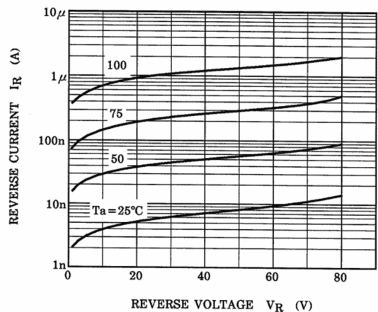
Fig. 7.2 I_R - V_R
