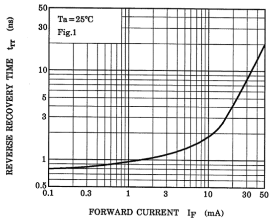
Fig. 7.4 t_{rr} - I_F
