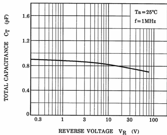
Fig. 7.3 C_t - V_R
