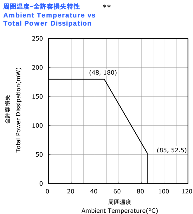
** 周囲温度-全許容損失特性
