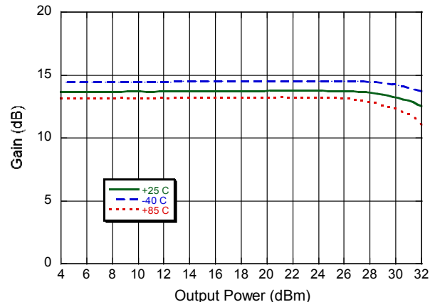
P1dB
