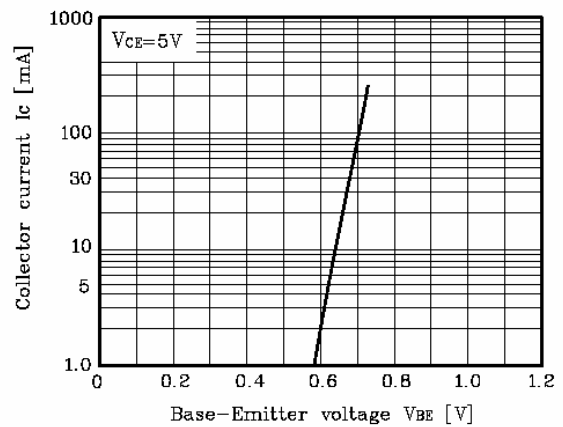
Fig. 2 I_C - V_{BE}
