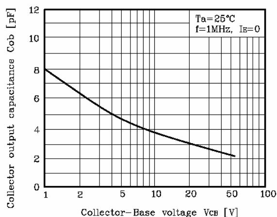
Fig. 5 C_{ob} - V_{CB}
